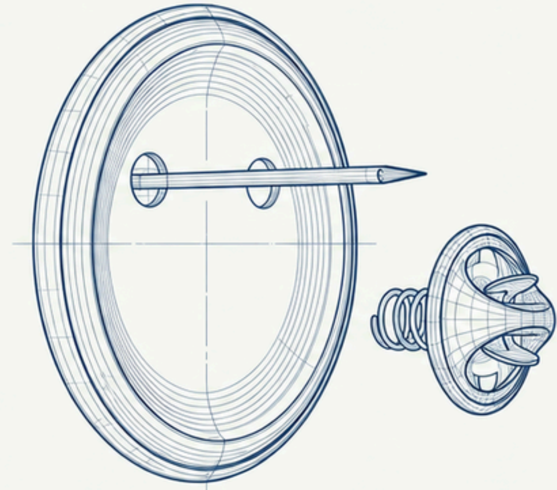
ASSEMBLAGE DU PIN - VUE ARRIÈRE
